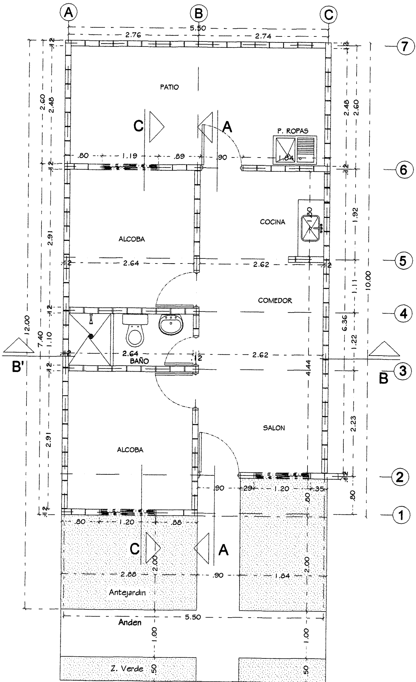
PLANTA CASA TIPO AREA 42M2
