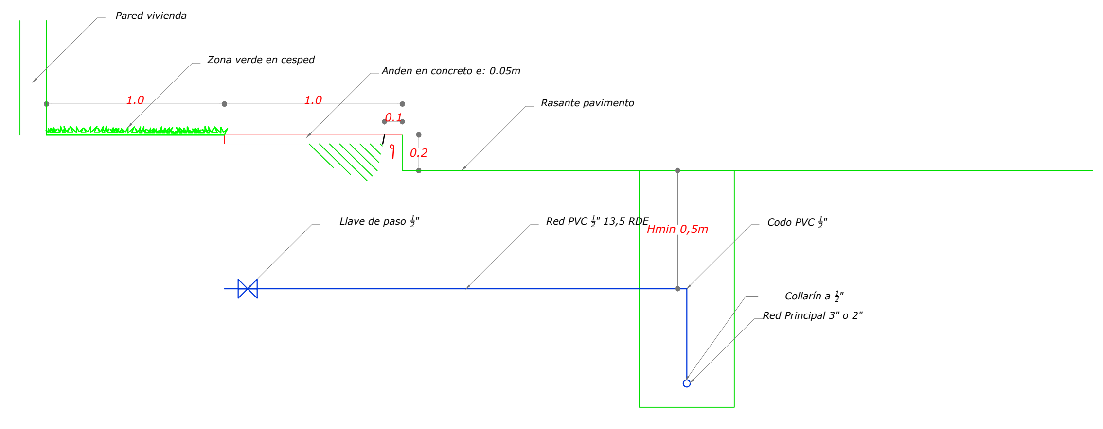
DETALLE CONEXION DOMICILIARIA ESCALA 1:5
