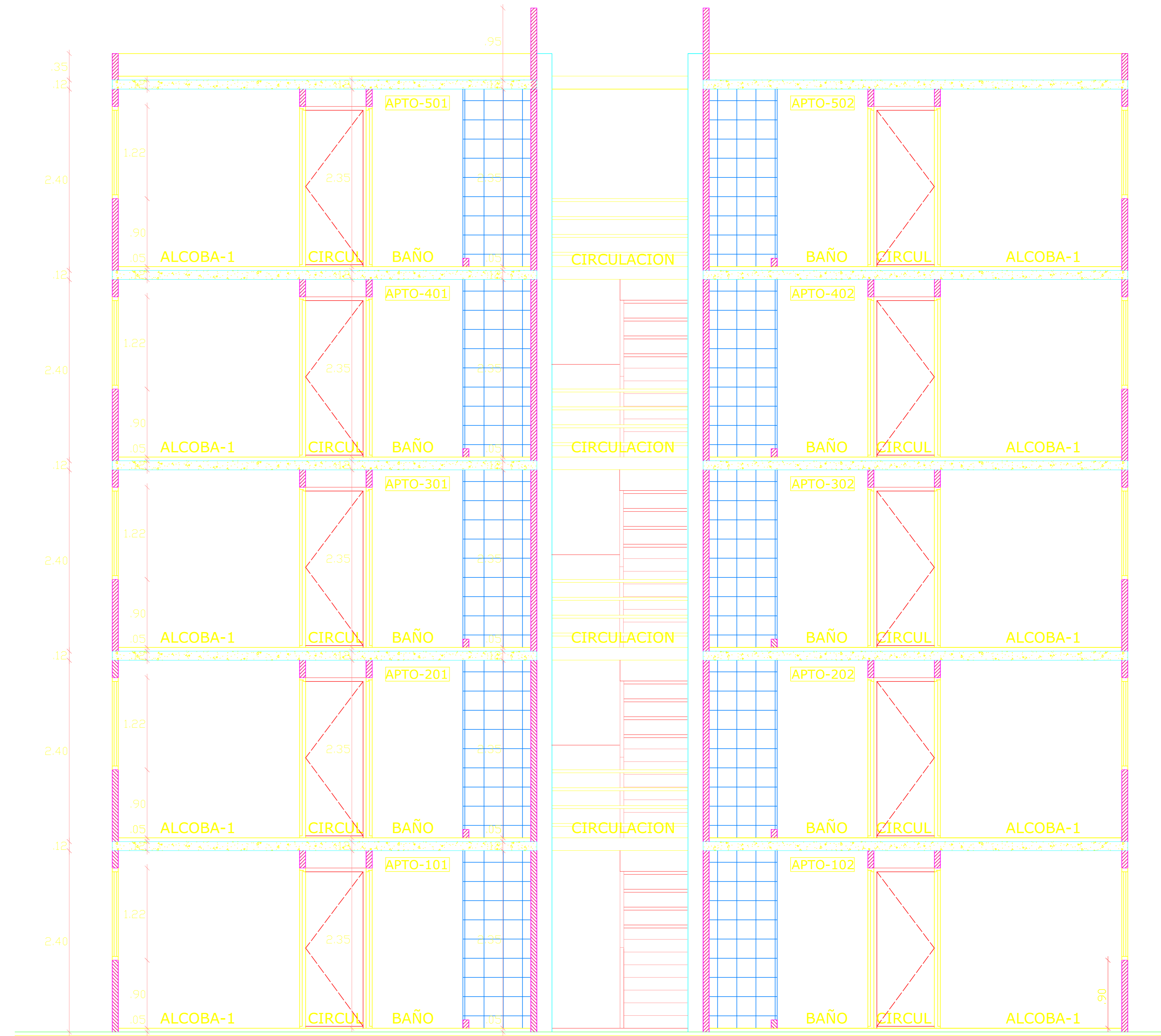
CORTE B, B'
