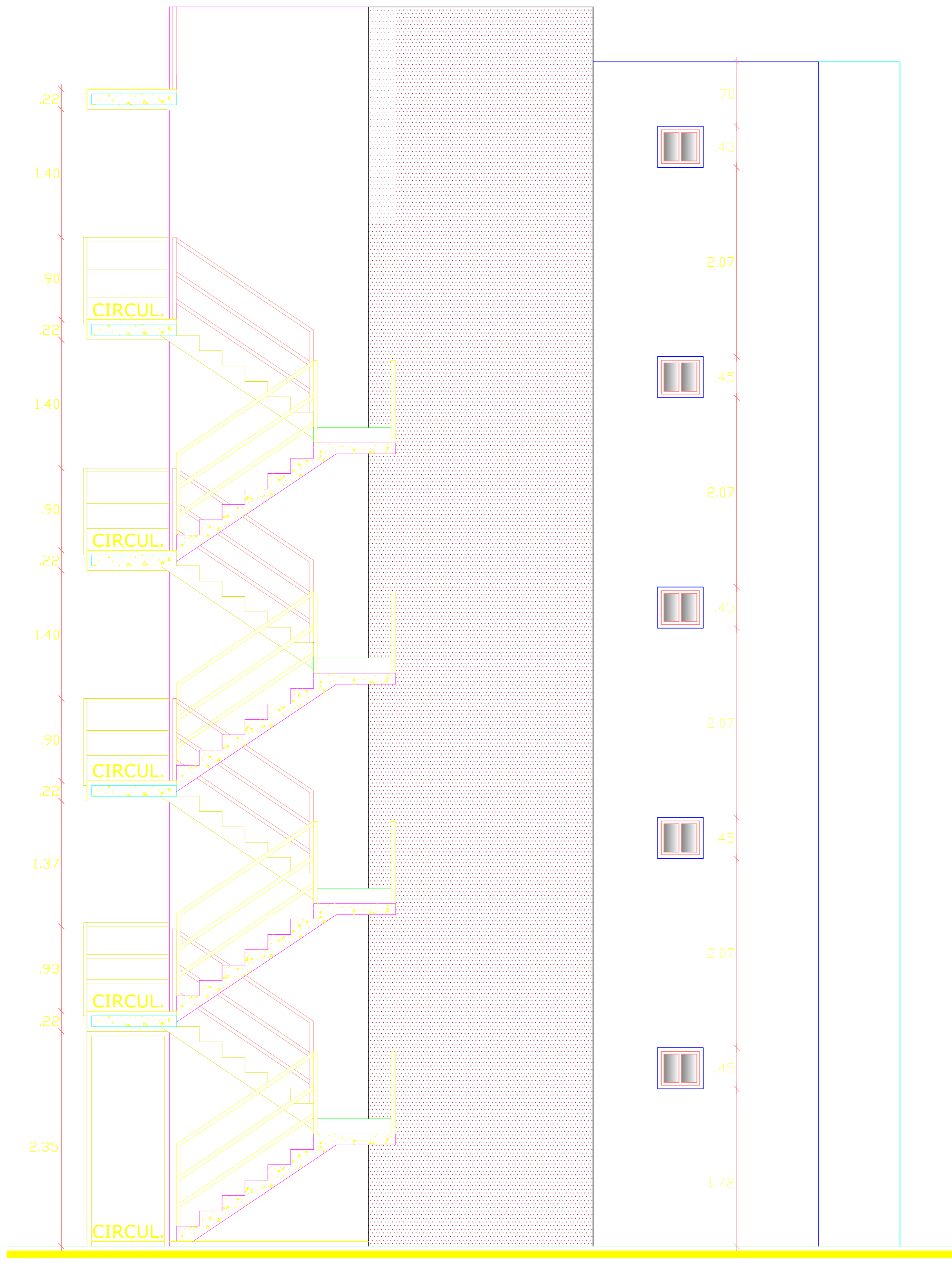
CORTE-FACHADA ESC. __ 1:50
