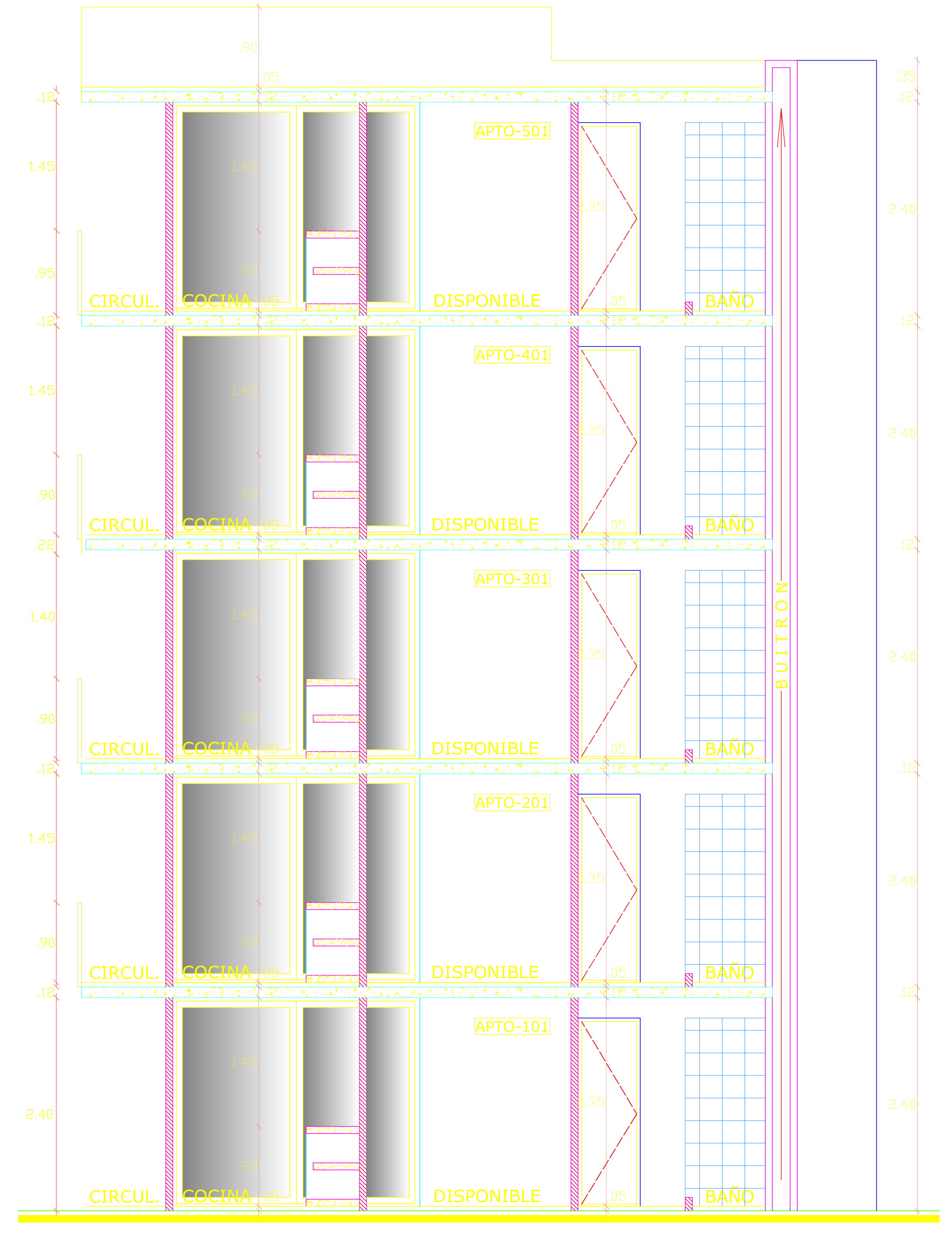
CORTE-A,A' ESC. __ 1:50
