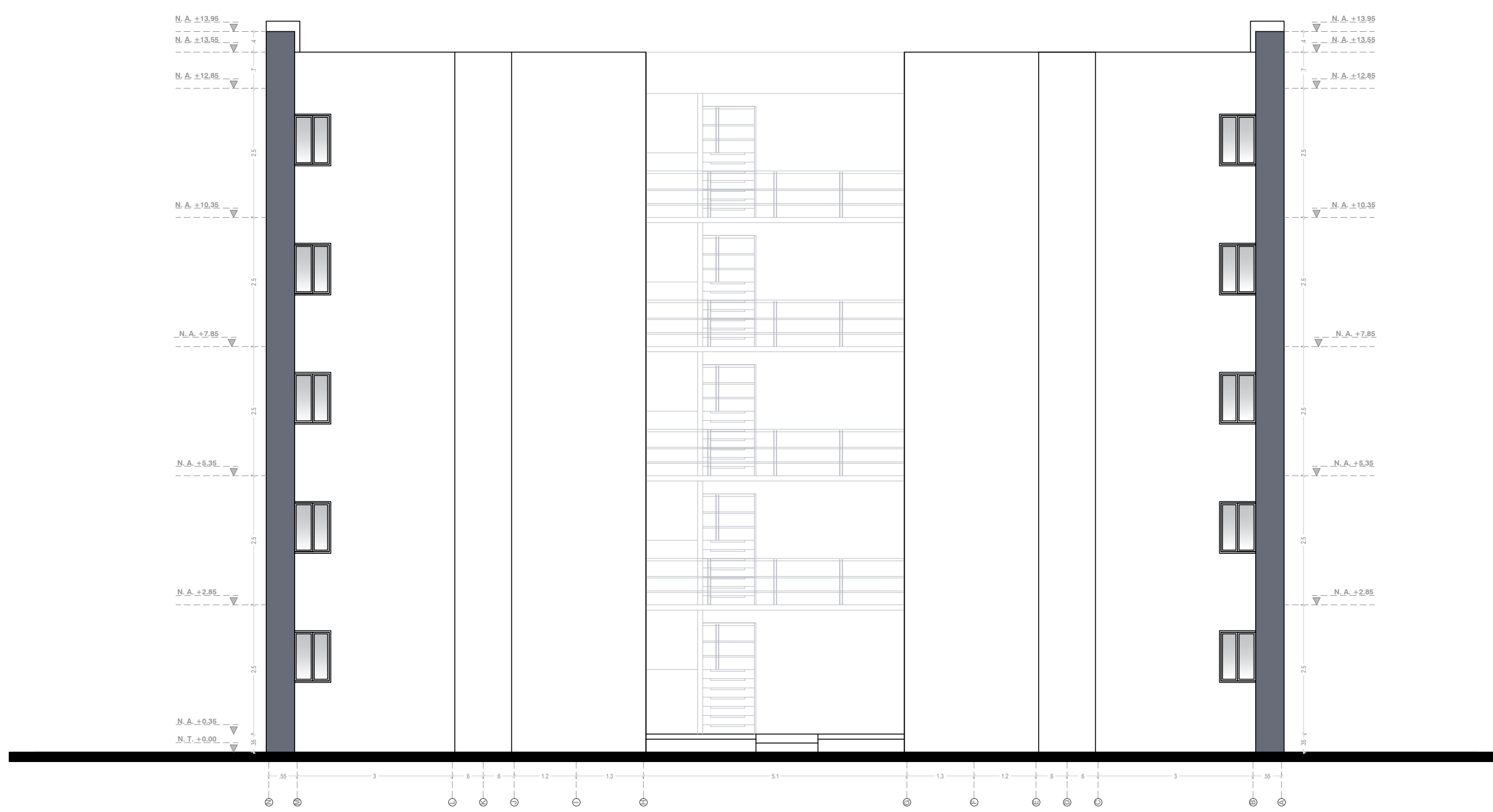
FACHADA LATERAL 1er A 5to - NIVEL
