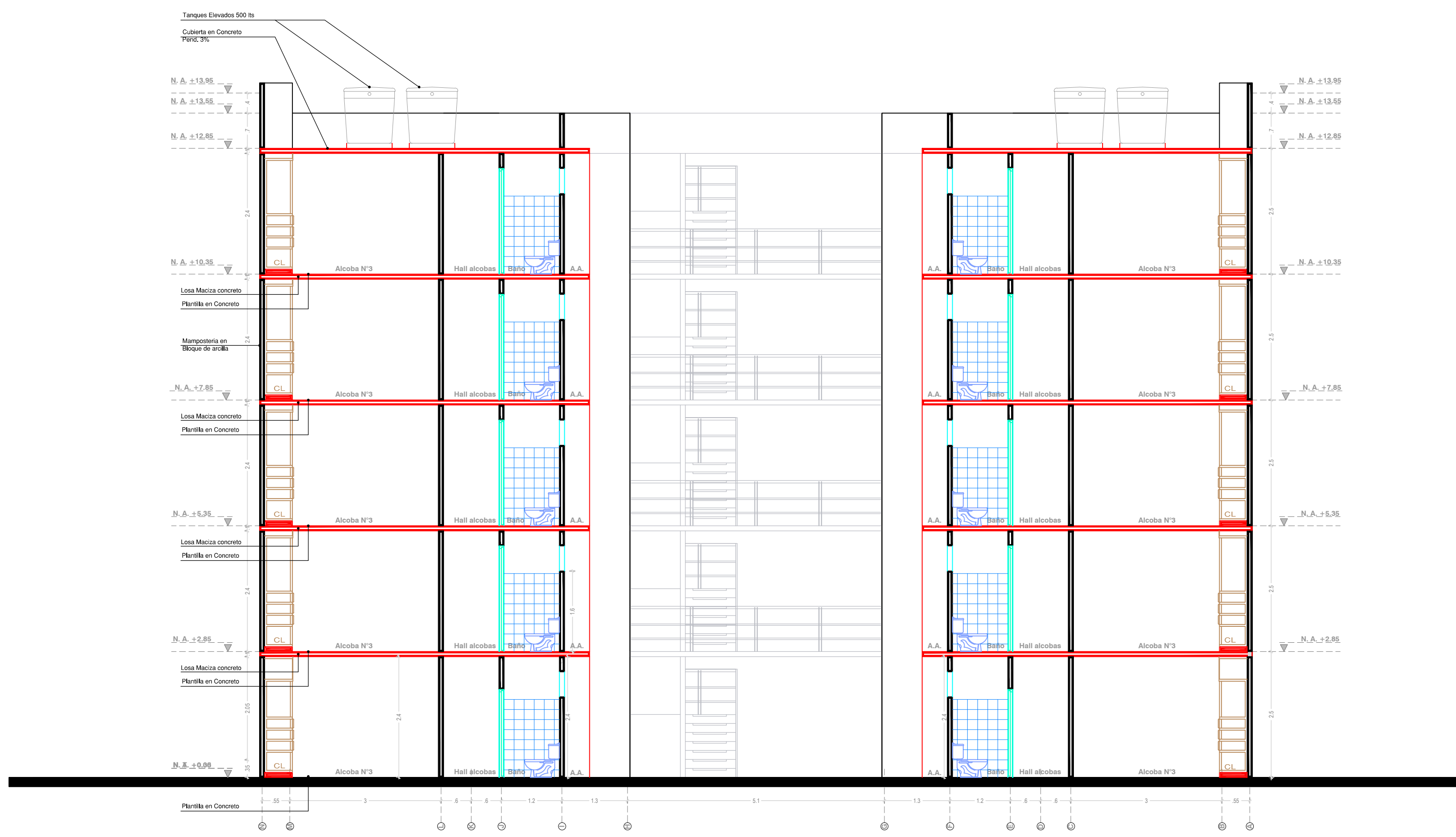
CORTE TRANSVERSAL TORRE TIPO APTOS 1er A 5to - NIVEL
