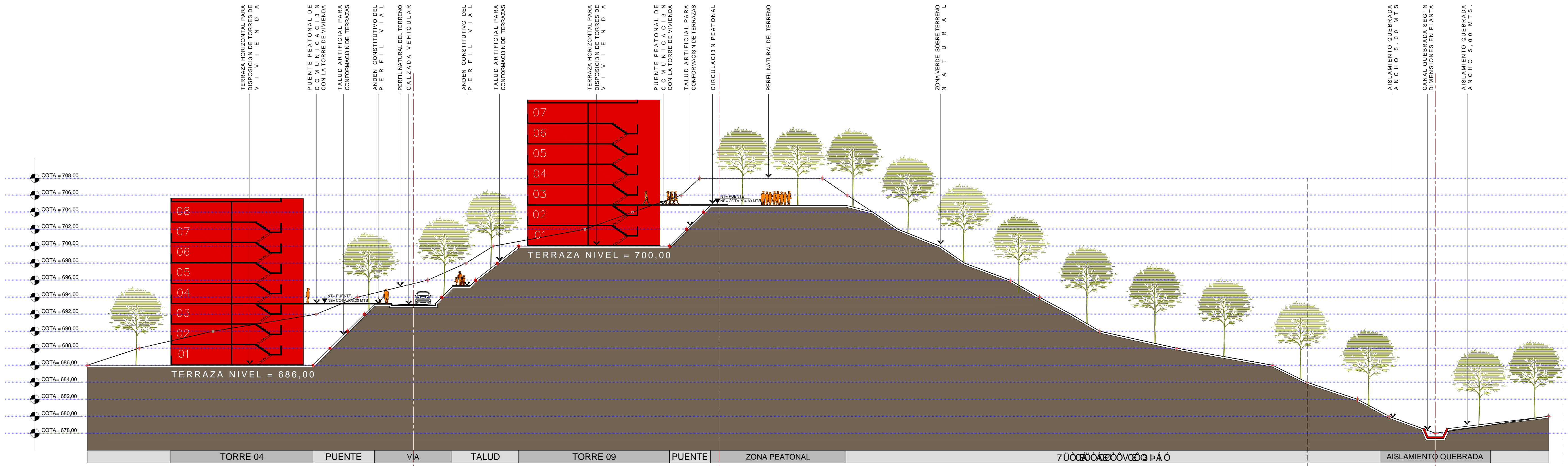
01 PERFIL URBANO A-A' ESCALA 1: 250
